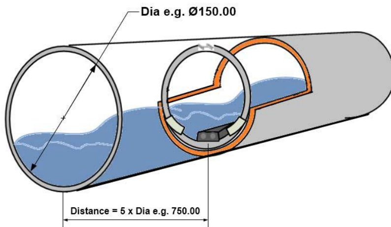
Требуемое расстояние в 5 диаметров от отверстия трубы
