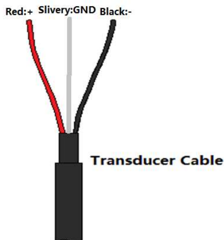
Рис. 2.4 Кабель датчика
