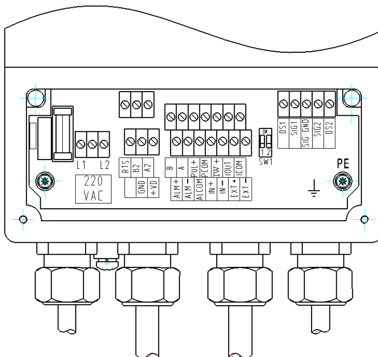
Рисунок 33. Клеммная колодка раздельного типа (ВП – RB101)
