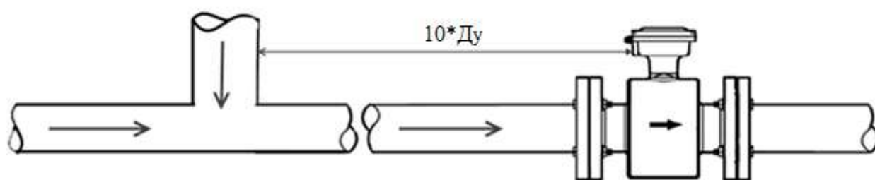
Рисунок 12. Расстояние от точки смешивания потоков
