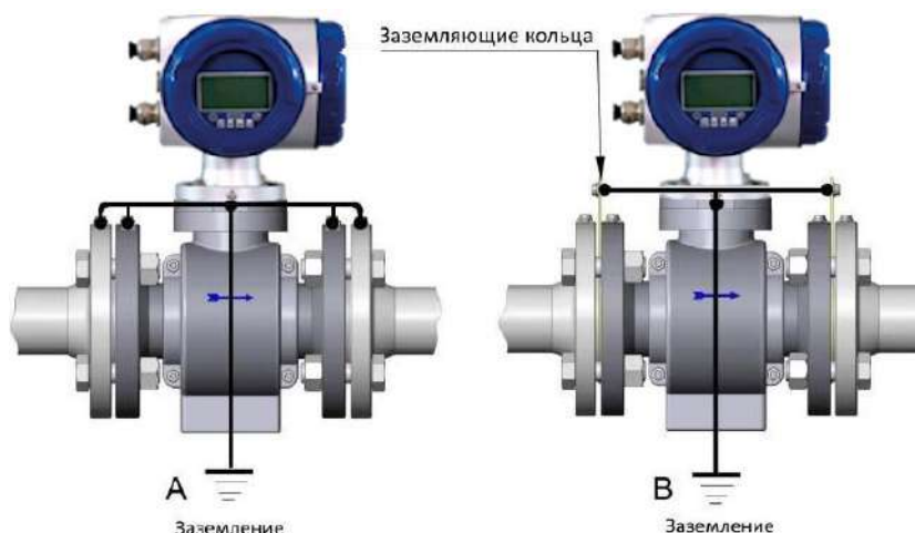
Рисунок 16. Варианты заземления расходомера
