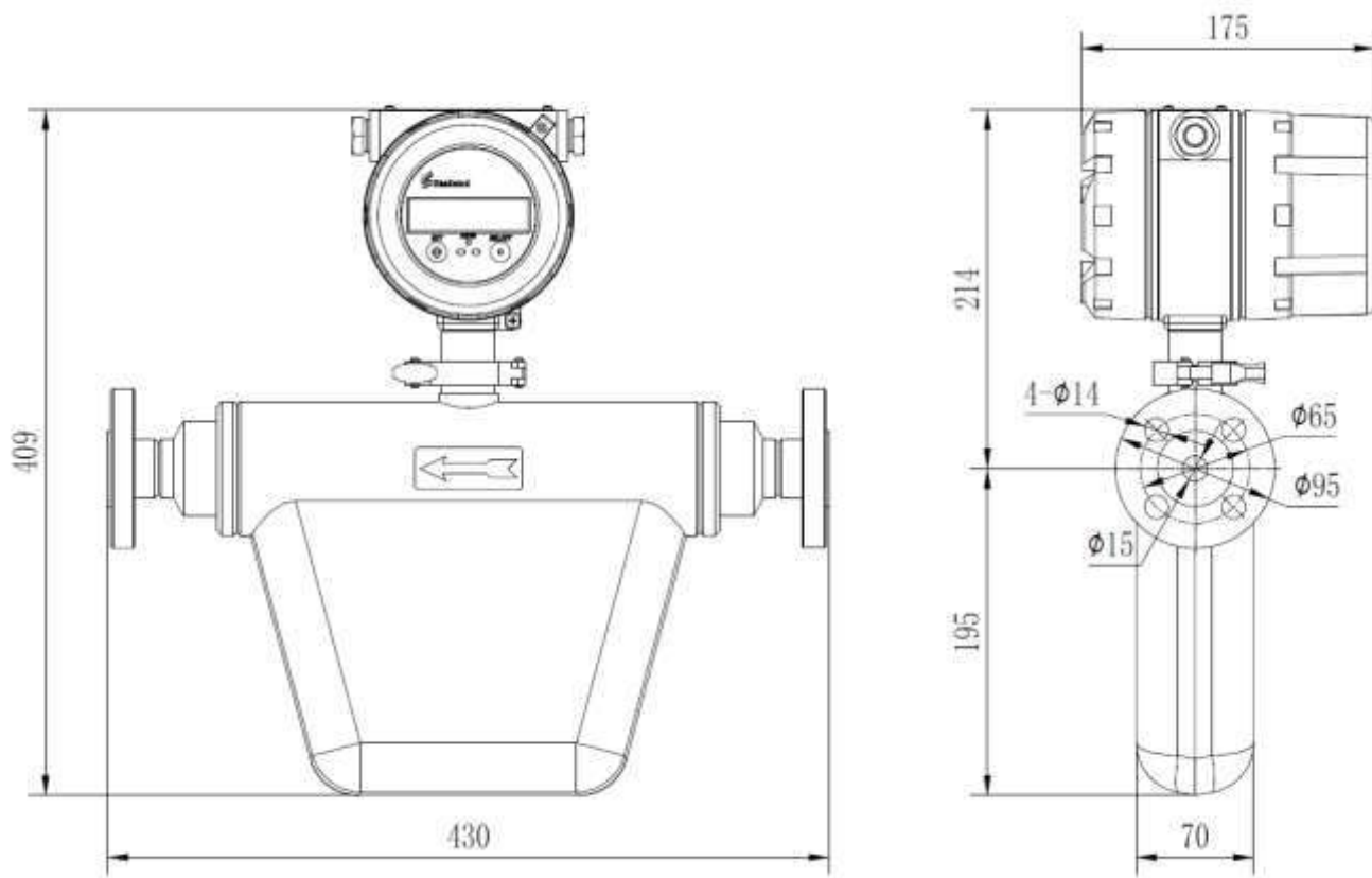
Чертёж Ду-15
