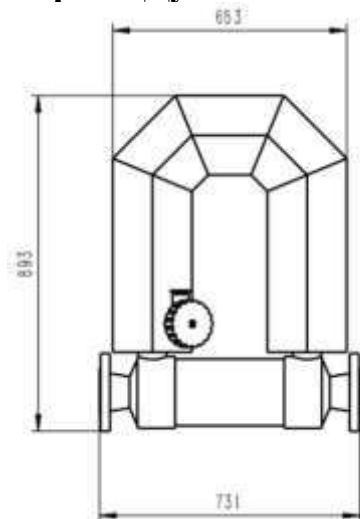
Чертёж Ду-80
