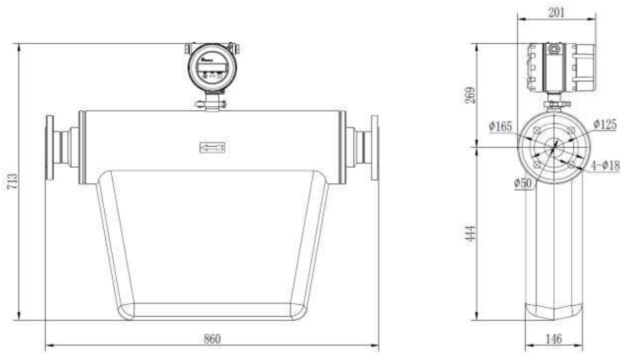
Чертёж Ду-50
