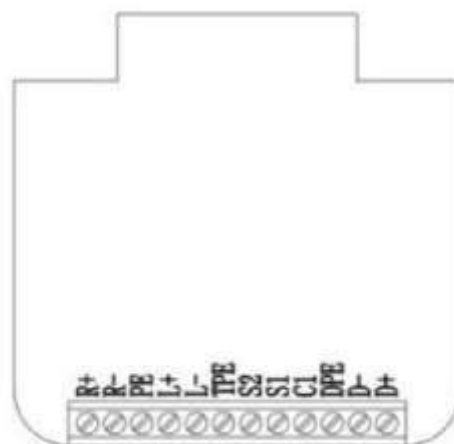
Рисунок 12. Клеммная колодка преобразователя сигнала
