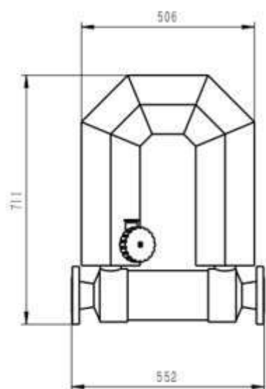
Чертёж Ду-50
