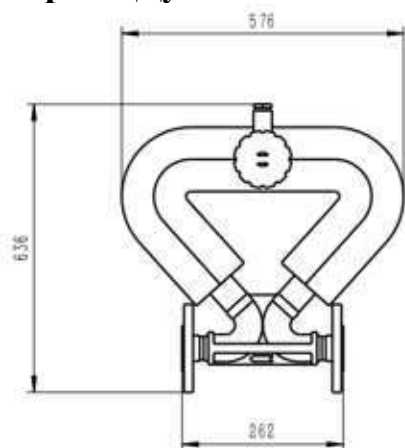
Чертёж Ду-40
