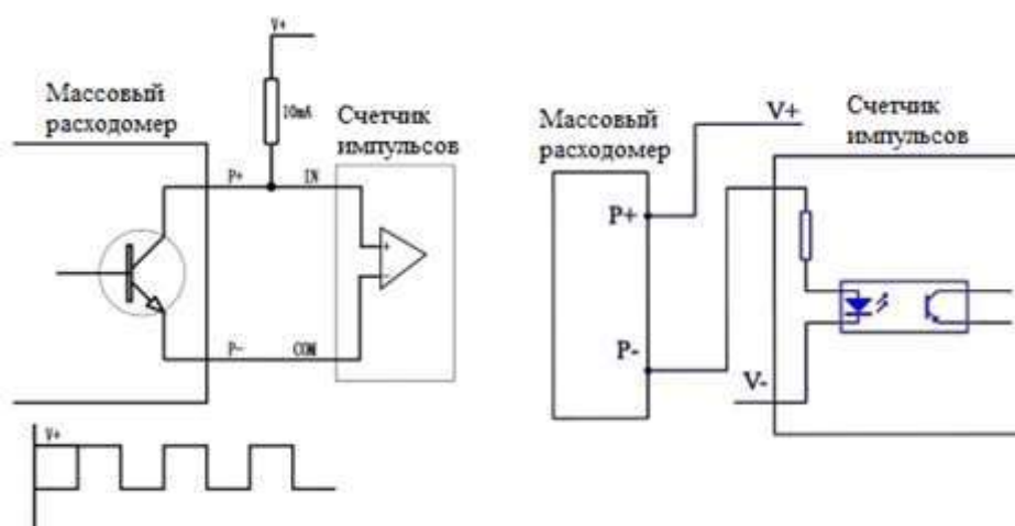
Рисунок 14. Схема подключения расходомера и приемника импульсов
