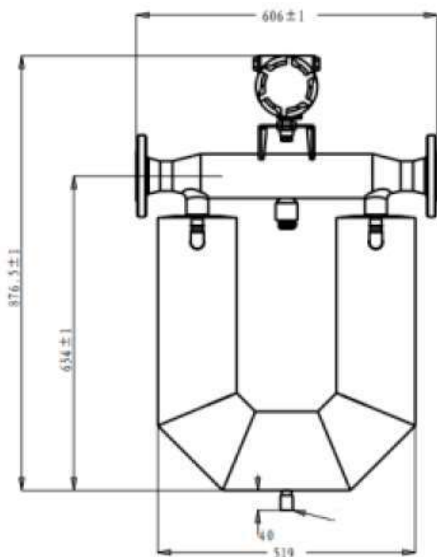
Чертёж Ду-80 с рубашкой
