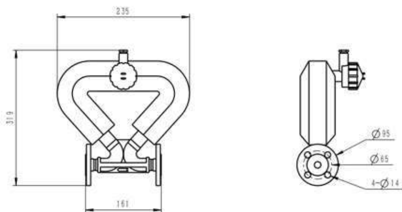
Чертёж Ду-6
