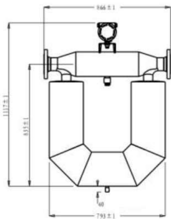
Чертёж Ду-80 с рубашкой
