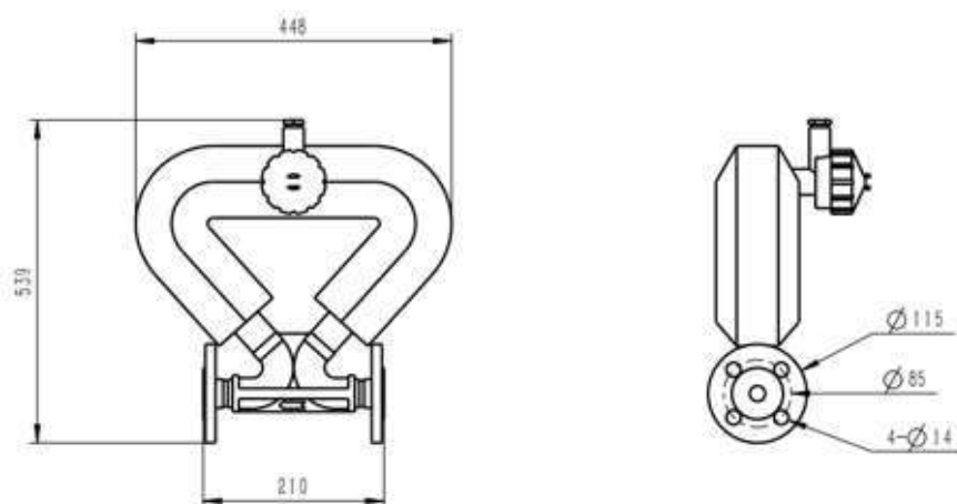
Чертёж Ду-25
