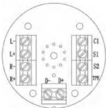
Рисунок 11. Клеммная колодка датчика
