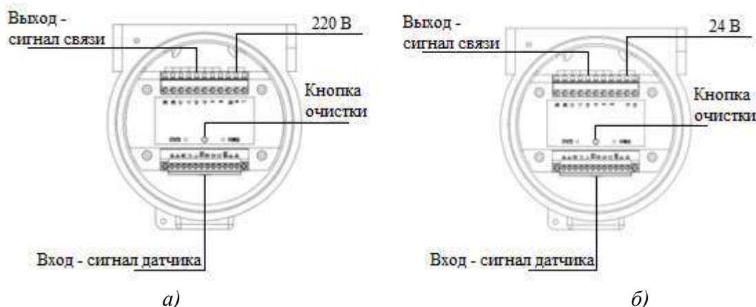
Рисунок 15. Коммутационные панели
