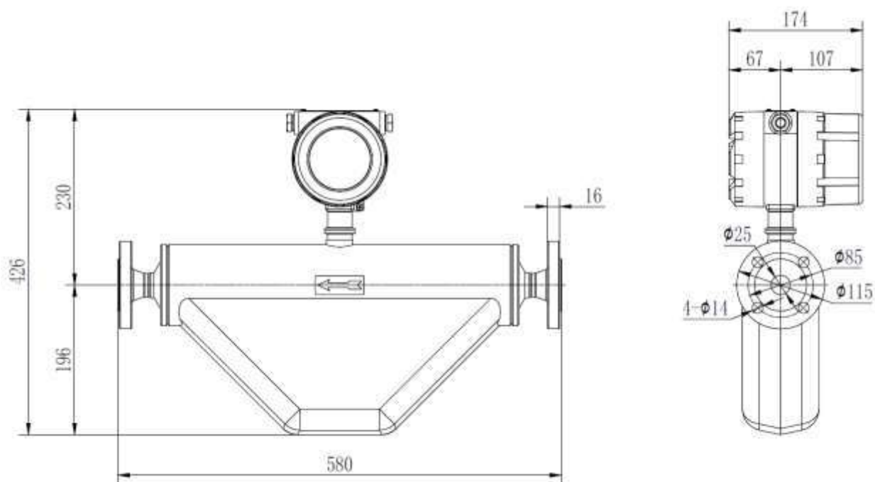
Чертёж Ду-25
